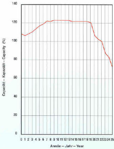
Capacité – Kapazität – Capacity
