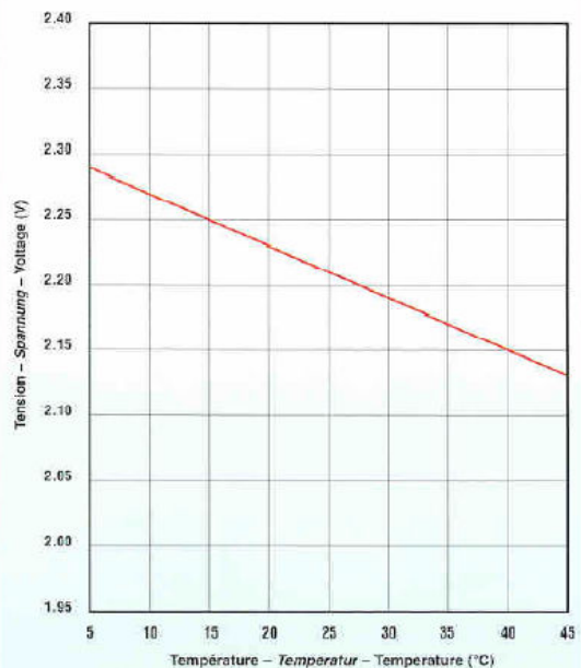
Tension flottante – Schwebespannung Float Voltage
