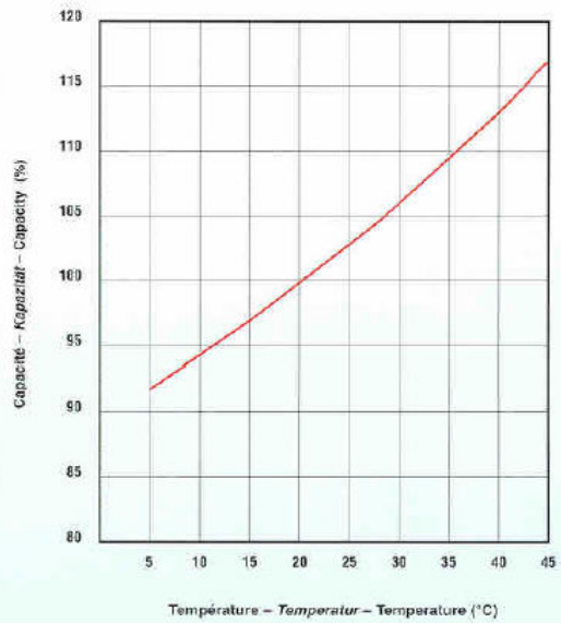
Capacité/Température – Kapazität/Temperatur Capacity/Temperature
